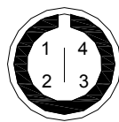
Pinout connettore Binder 719 4 pin femmina vista lato saldatura
