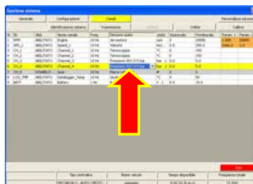
Figura 35: Race Studio 2 – Finestra canali in ingresso.
