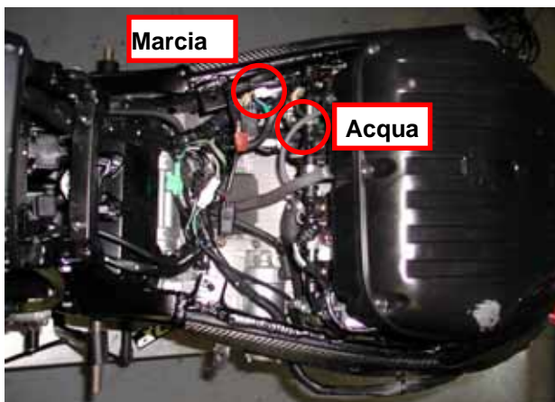
Figura 17: connettori di serie –temperatura dell'acqua/ cambio
