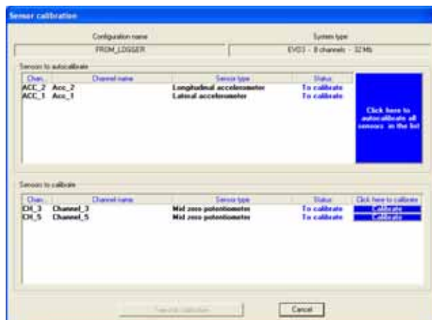
Figura 36: Race Studio 2 – Schermata di Calibrazione
