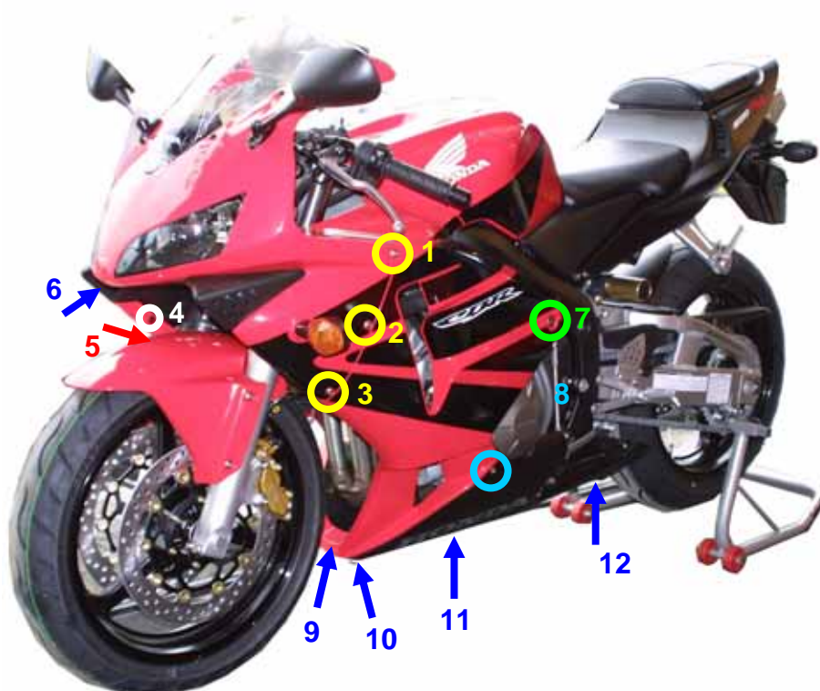
Figura 5: Posizione di tutte le viti laterali e frontali della moto.
