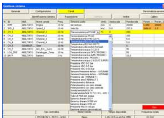
Figura 33: Race Studio 2 – Finestra canali - Gold
