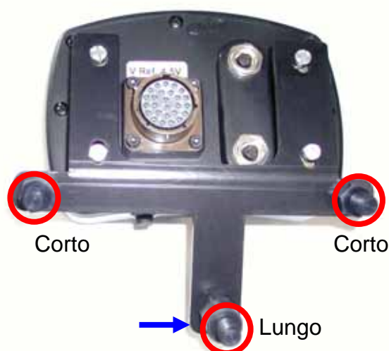
Figura 23: I perni di fissaggio della staffa
