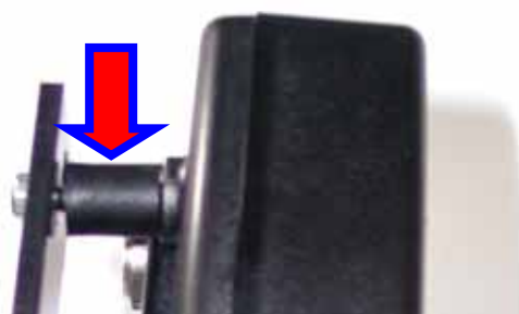
Figura 21: montanti anti-vibrazione – particolare
