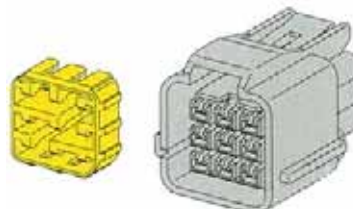
Figura 4: connettore Furukawa femmina a 9 pin.
