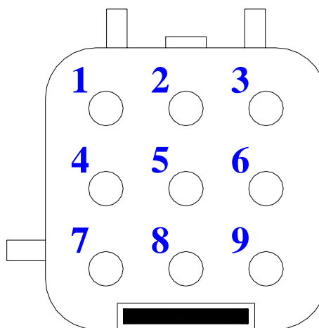
Figura 5: MXL PRO 05 connettore Furukawa maschio.
