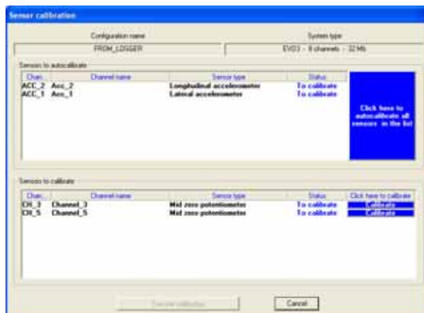
Figura 11: Race Studio 2 – Finestra di Calibrazione
