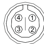
Pinout connettore Binder 719 - 4 pin maschio: vista lato terminazioni di saldatura
